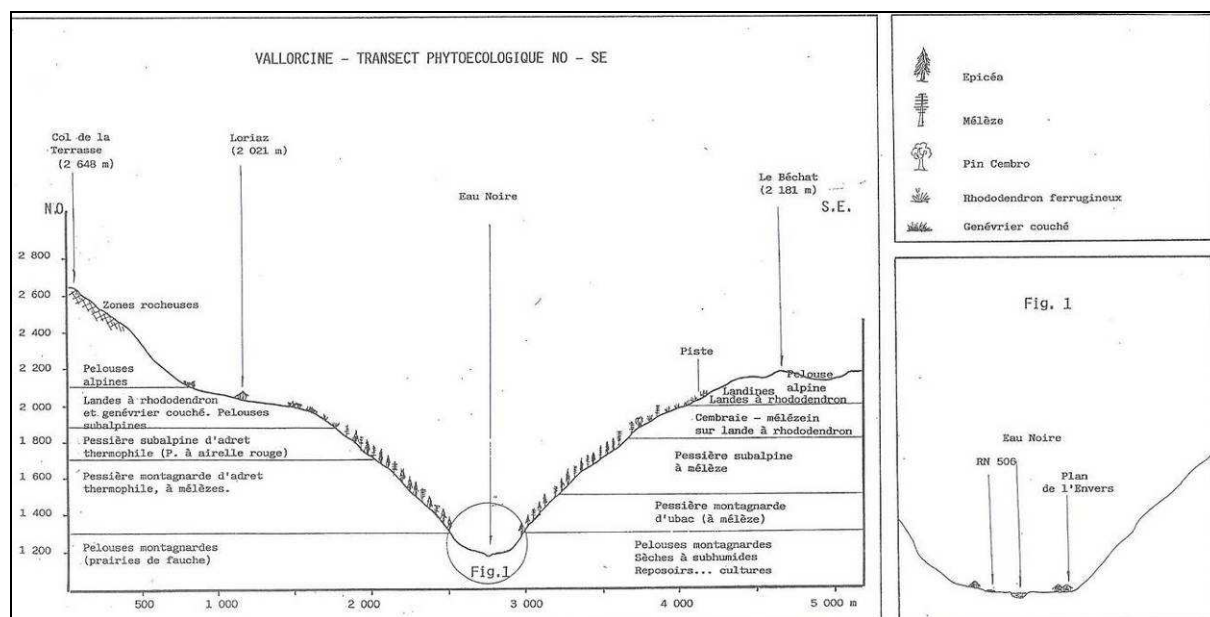
Figure 1: Transect phytoécologique de la vallée de Vallorcine (Plan de révision d'aménagement forestier 2009-2023. Forêt communale de Vallorcine)
